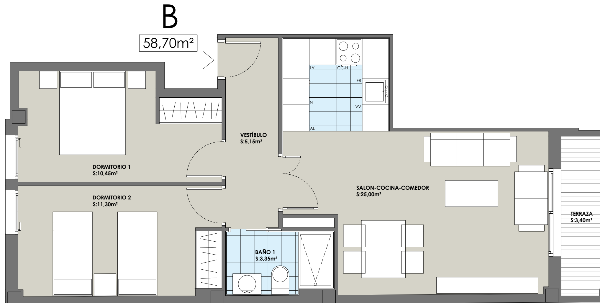
PLANTA 6ª
