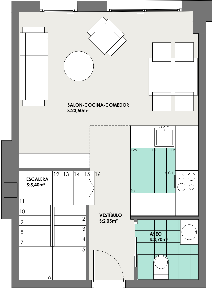
PLANTA 1ª (DUPLEX)
