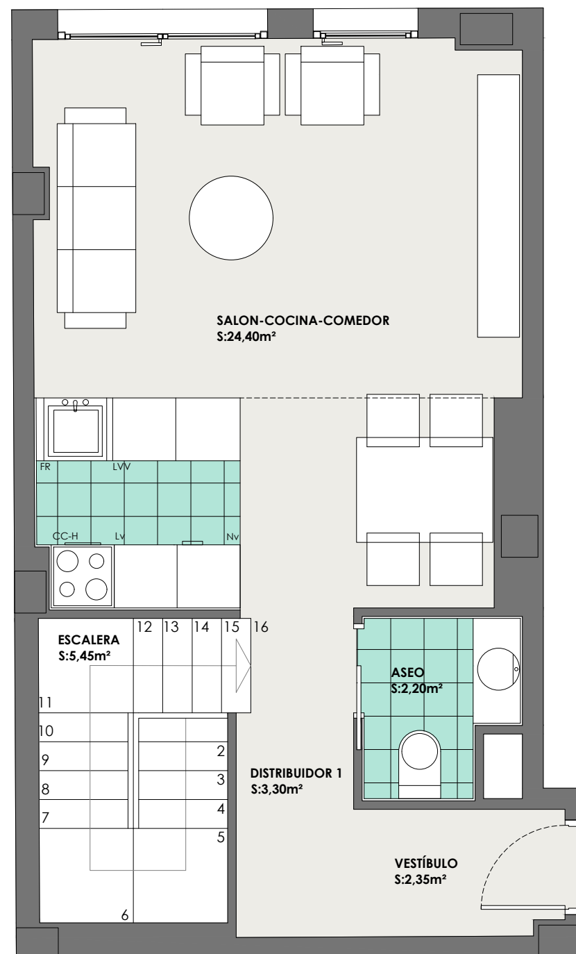
PLANTA 1ª (DUPLEX)
